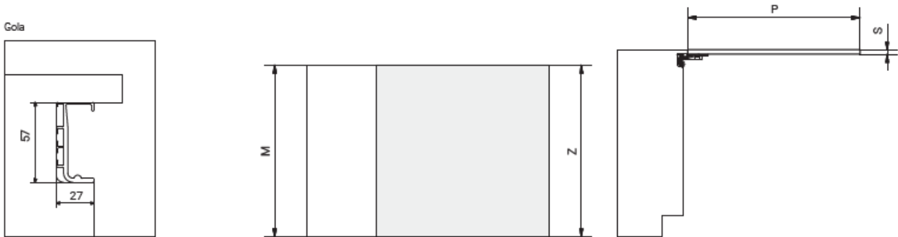
Dinamico PROFILO GOLA + STAFFE GOLA PROFILE + BRACKETS
